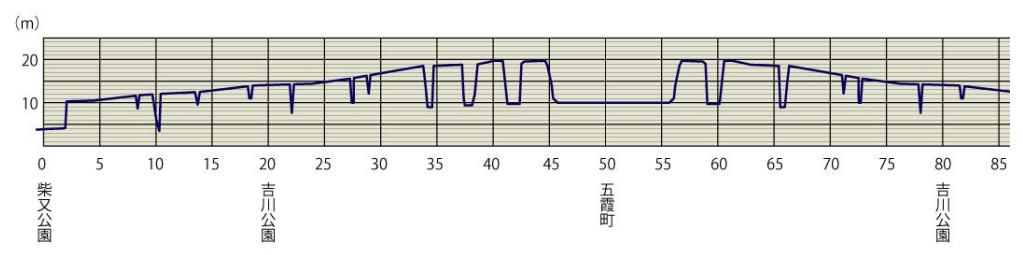
【柴又 100K】 100km コース高低図 2018
